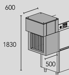
DR24 4,5 kW Asciugatura
