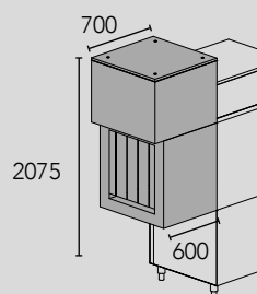
DR64 4,5 kW Elettrico DR69 9 kW Elettrico Asciugatura
