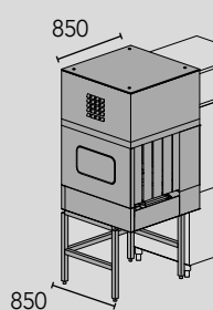
DRA94MC 4,5 kW Elettrico DRA99MC 9 kW Elettrico Asciugatura su curva meccanizzata 90° da utilizzare soltanto con cesti originali DIHR
