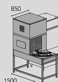
DRA184MC 4,5 kW Elettrico DRA189MC 9 kW Elettrico Asciugatura su curva meccanizzata 180° da utilizzare soltanto con cesti originali DIHR
